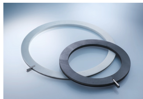
Dichtringe der Baureihe Espey® WD200 (3-teilig, stumpfer Stoß) – Kohle/PTFE-Compound
