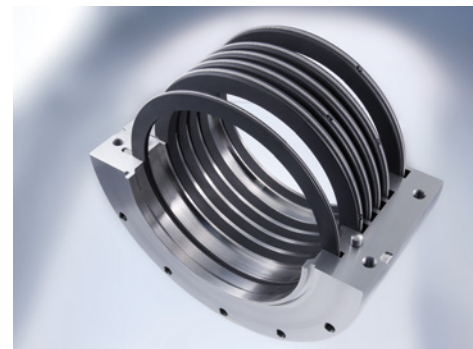
Espey® WD200/500: obere Gehäusehälfte demontiert
